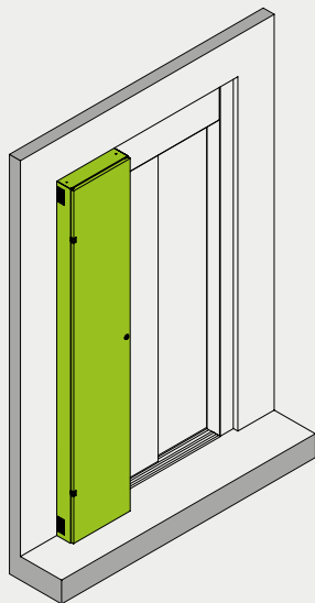
FIANCO PORTA AUTOMATICA 1 L420 x P210 x H2238
