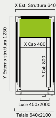
SENZA PORTA Testata minima 2600m
