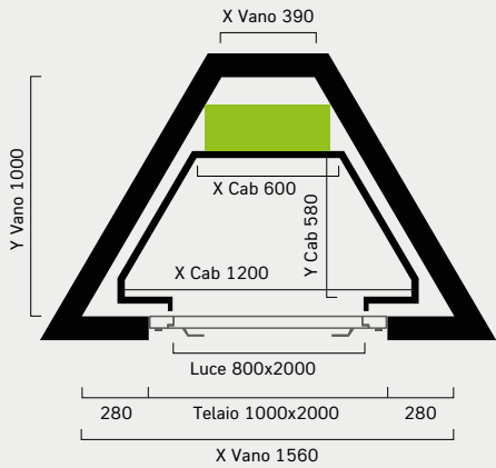
TRAPEZODALE Testata minima 2600m
