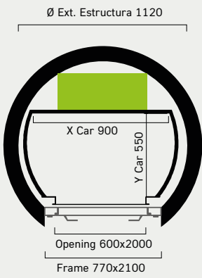
TONDO Testata minima 2600m
