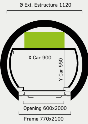
TONDO Testata minima 2600m
