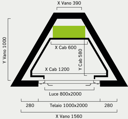
TRAPEZODALE Testata minima 2600m
