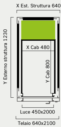
SENZA PORTA Testata minima 2600m
